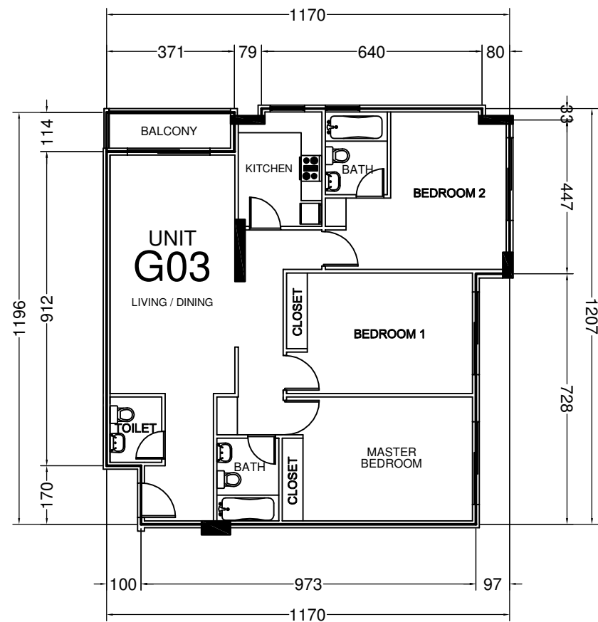
UNIT LAYOUT SCALE: NTS
